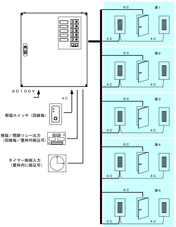
〈ブロック図〉
