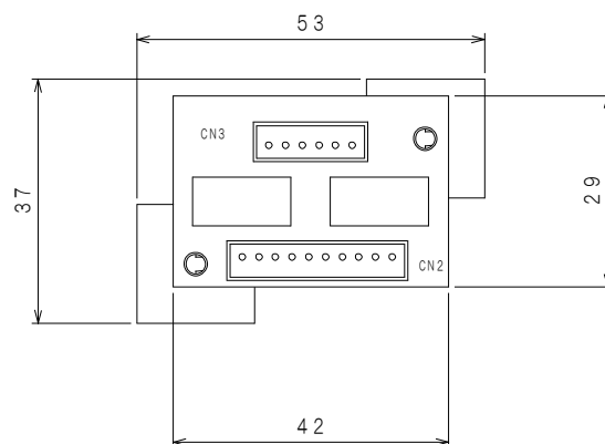
【外形寸法図】
